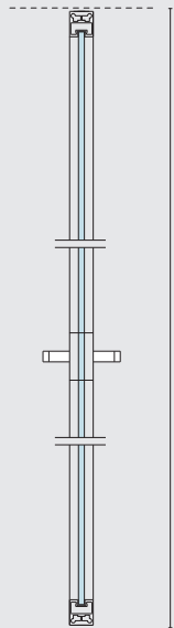
Taatsdeur zonder kozijn Pivot door without frame
