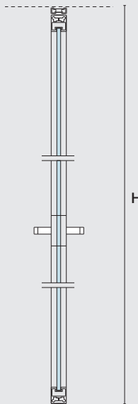
Taatsdeur met kozijn Pivot door with frame
